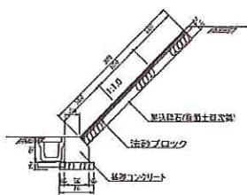
断面図 S=1:3.0
