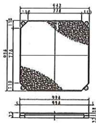
A形ブロック 998×998×70 参考重量 161kg
